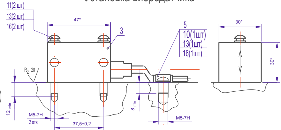
Установка вибродатчика
