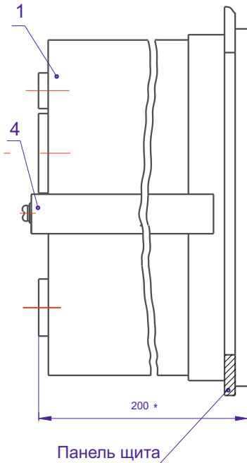
УСТАНОВКА БЛОКА
