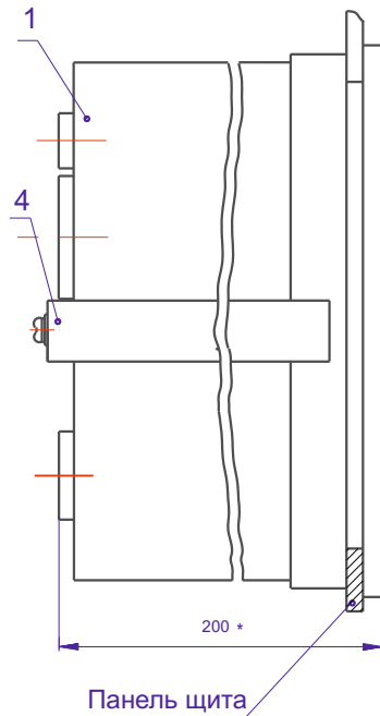
УСТАНОВКА БЛОКА
