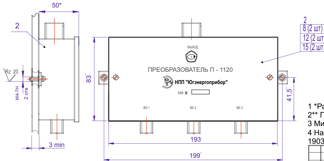
Установка преобразователя
