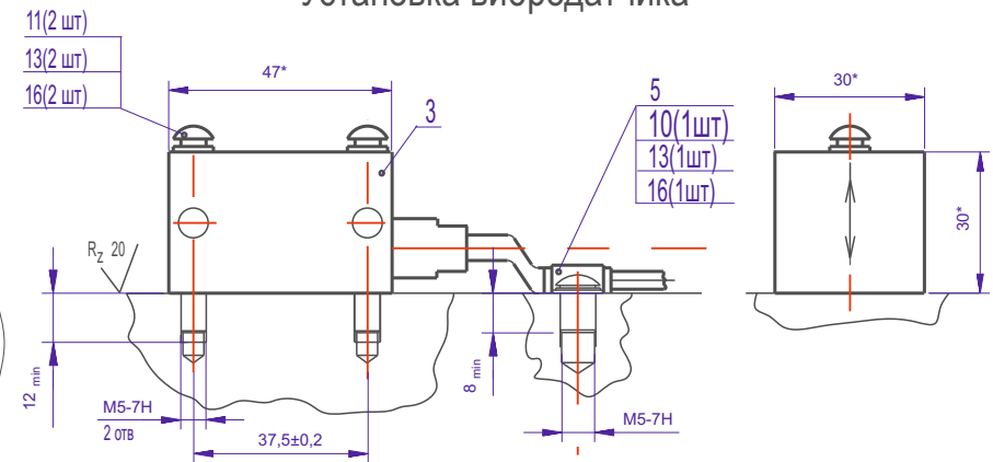
Установка вибродатчика
