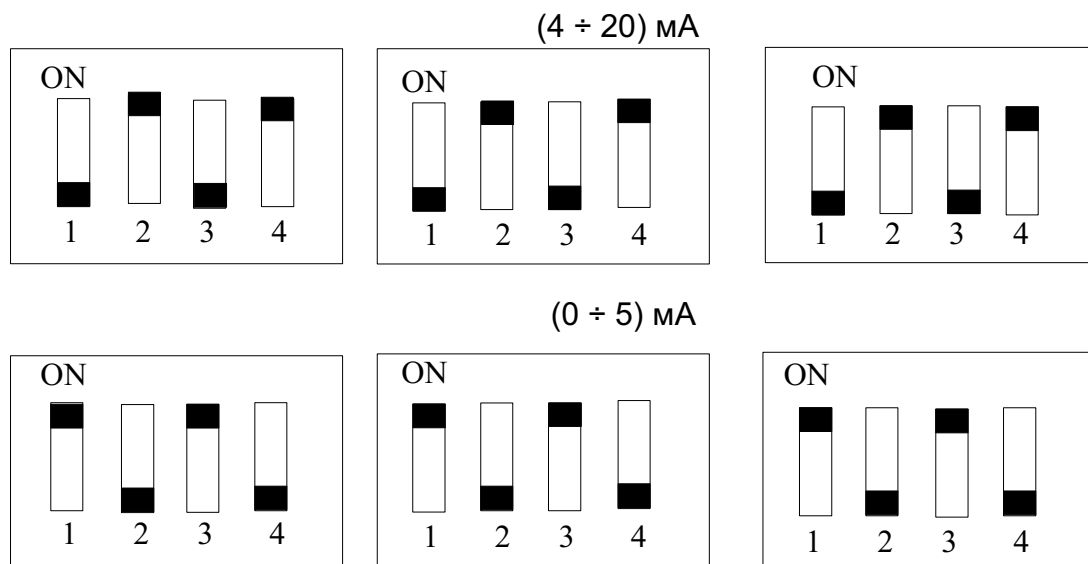
Положение DIP-переключателей
